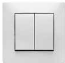
DOBLE CONMUTADOR De empotrar. 10 A. 250 V. color blanco. 4,20 Ref. 83.220
